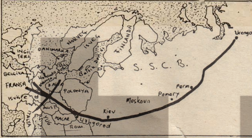
Tartışmalara neden olan Sovyet-Avrupa doğal gaz boru hattı.
